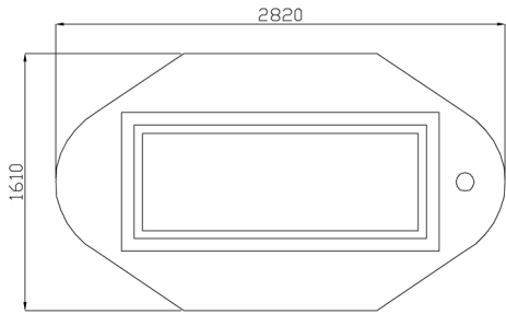
Lid Plan
