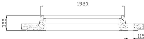
Lid Section
